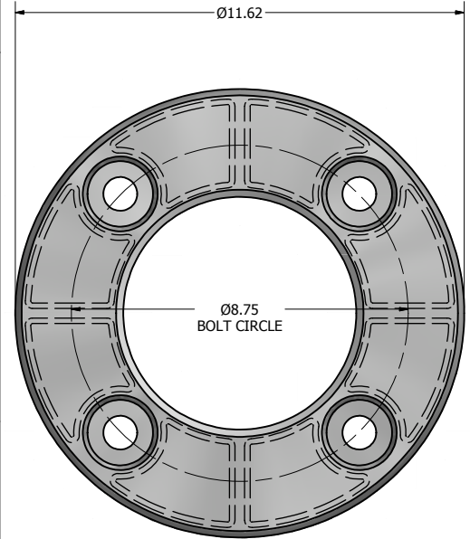
Ø11.62 X 1.88 THK. BASE CASTING
